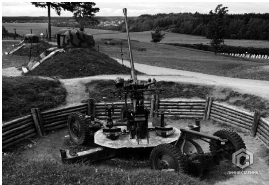
Зенитная пушка 61-К.
